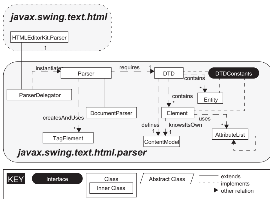
Figure 2-2. HTMLEditorKit 's parser class diagram.
